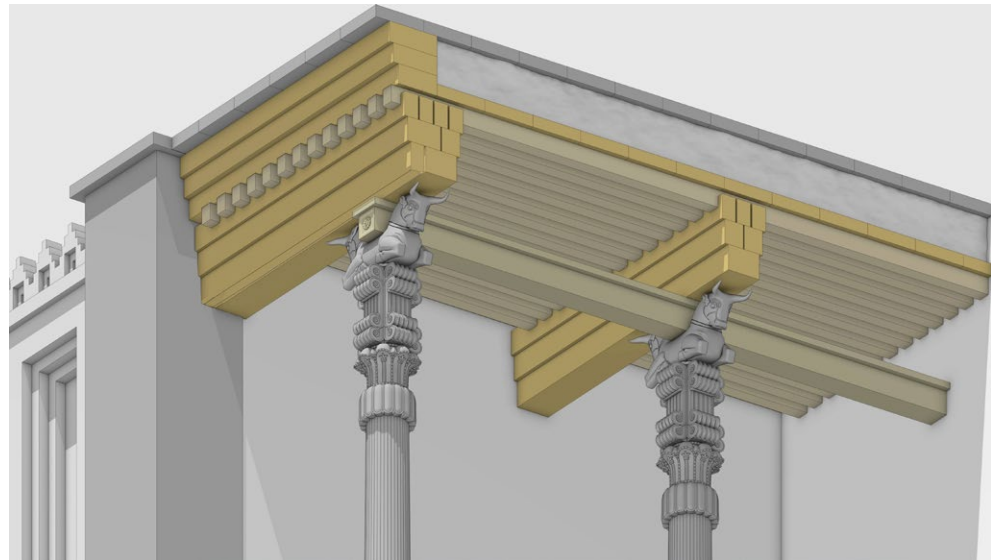
تصویر ۱۳: جزئیات عناصر پوشش‌دهنده، پیش‌آمدگی و اتصالات سقف در ایوان کاخ‌ها (منبع Motamedmanesh 2022, 309). تغییرات توسط نویسنده
