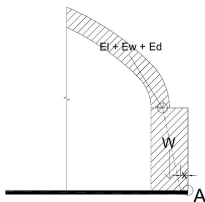
تصویر ۲۰: نیروهای وارد بر تکیه‌گاه طاق
