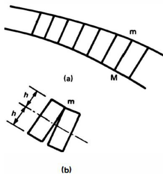
تصویر ۱۱: تشکیل مفصلی میان دو بلوک از مصالح بنایی (Heyman 1995)
