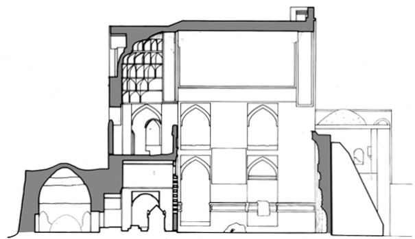
تصویر ۵: مقطع ب-ب (آرشیو میراث فرهنگی، صنایع دستی و گردشگری اصفهان، درخواست شده توسط گروه ISMEO، ۱۳۵۲ش)
