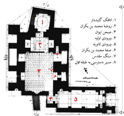
تصویر ۳: پلان بنای پیربکران (آرشیو میراث فرهنگی، صنایع دستی و گردشگری اصفهان، درخواست‌شده توسط گروه ISMEO، ۱۳۵۲ ش، افزوده‌ها از نویسندگان)
