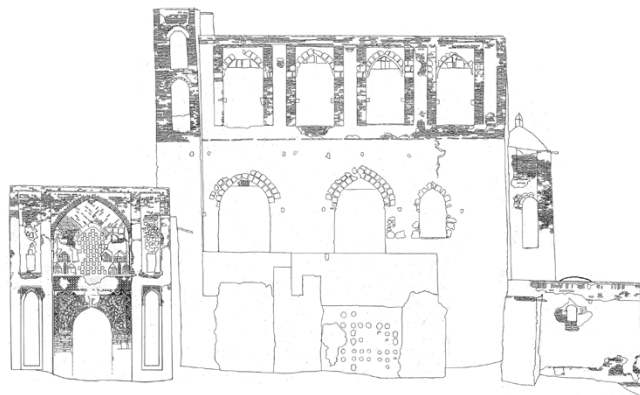
تصویر ۶: نمای شرقی (ج-ج) (آرشیو میراث فرهنگی، صنایع دستی و گردشگری اصفهان، درخواست شده توسط گروه ISMEO، ۱۳۵۲ش)
