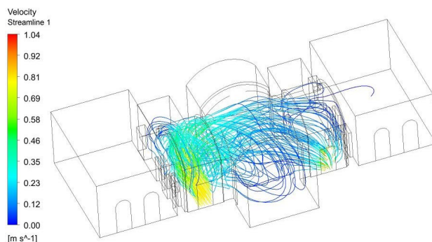
تصویر ۷: الگوی جریان هوا در حالت وضعیت موجود بازشوها
