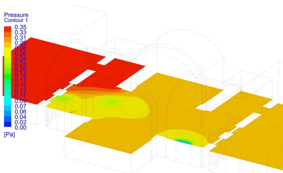
تصویر ۸: پلان فشار نسبی در یک ارتفاع نمونه ( 1/2 متر از کف)
