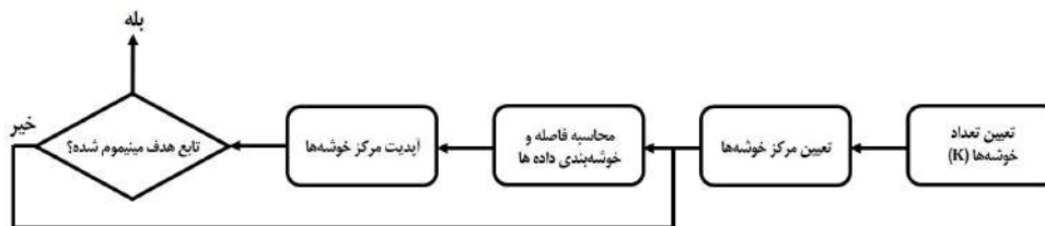
تصویر ۸: عملکرد الگوریتم k-means (Howsam 2022)
