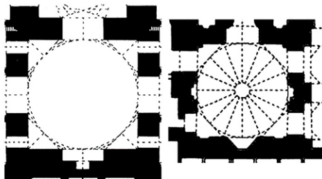
تصویر ۵: ساختار دو نمونه مرسوم گنبدخانه در سنت معماری ایران؛ گنبد مسجد جامع اردستان (راست)؛ گنبدخانه مسجد جامع عباسی (چپ) (حاجی قاسمی ۱۳۸۳، ۳۶؛ ۱۳۷۵، ۳۴)
