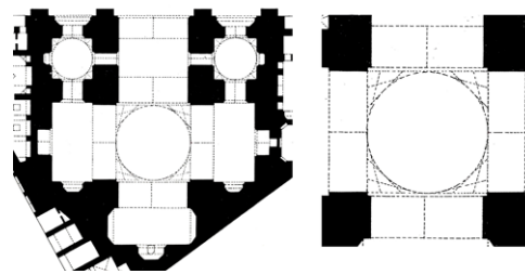
تصویر ۴: ساختار گنبدخانه مدرسه سپهسالار؛ به حداقل رسیدن جرزها در کناره‌ها برای گشودگی حداکثر گنبدخانه به اطراف در این طرح مشهود است (حاجی قاسمی ۱۳۷۷، ۹۶).
