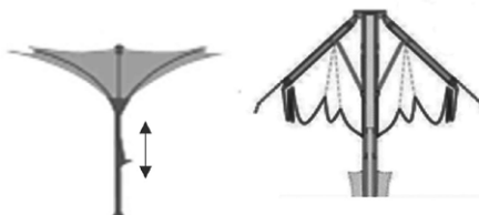
تصویر ۱۱: راست: مکانیزم حرکتی چتری رو به پایین، چپ: مکانیزم حرکتی چتری رو به بالا (Hemmerling 2017)
