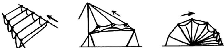
تصویر ۲: مکانیزم حرکت غشایی، راست: حرکت دایره‌ای، میانه: حرکت مرکزی، چپ: حرکت خطی (Mollaert 1996)
