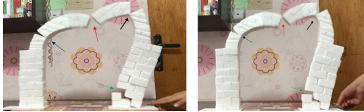
تصویر ۱۶: مکانیسمی با چهار ترک (تقریباً مشابه نشست) ناشی از اثر زلزله. راست: ترک‌های ناشی از ضربه. چپ: ترک در آغاز ربع سیکل اول ۳۳ در حرکت رفت‌وبرگشتی. مدل‌سازی، فیلم و عکس از دانشجو: فاطمه عرب‌پور، درس سیستم‌های ساختمانی، ۱۳۹۸
