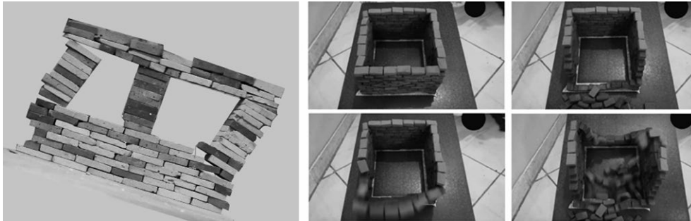
تصویر ۲۷: بررسی رفتار دیوارهای بنایی استفاده از روش دوران صفحه زمین. راست: بررسی شکست عمود بر صفحه. چپ: بررسی اثر بازشوها. مدل سازی، فیلم و عکس از دانشجویان: نازنین نایبالی، فاطمه مکی و نگین شرفی، درس روستا، ۱۳۹۹.
