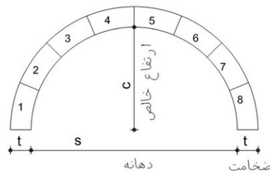
تصویر ۴: راست: هندسه قوس. چپ: آماده‌سازی قطعات قوس بدون چسباننده. اثر دانشجو: کیمیا افلاطونیان، درس سیستم‌های ساختمانی، ۱۳۹۸
