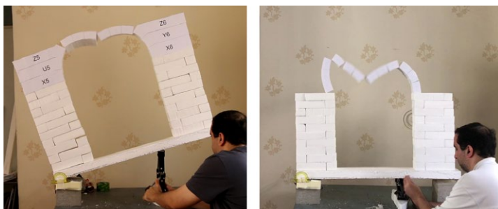
تصویر ۲۲: با ایجاد امکان اندازه‌گیری دقیق از طریق روش دوران صفحه زمین، دانشجو باید به بررسی اثرات تناسب هندسی سازه بر روی میزان پایداری لرزه‌ای آن بپردازد. مقایسه پایداری لرزه‌ای مجموعه در دو تناسب مختلف در اینجا مشاهده می‌شود: تغییر معنادر در پایداری لرزه‌ای سازه با تغییر مناسب در هندسه.
