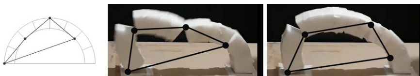
تصویر ۲۴: مسائل پیچیده‌تری چون محل متفاوت مفاصل‌ها در مدل تجربی نسبت به مدل نظری (تصویر ۲۳) در رفتار قوس ظهور می‌نماید؛ درحالی‌که محل مفاصل در مدل تصویر وسط بر مدل نظری منطبق است، در مدل تصویر راست، محل مفاصل‌ها تغییر کرده است.
