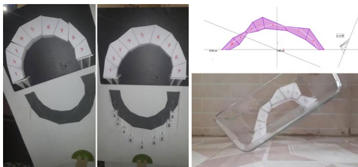
تصویر ۲۹: مراحل طراحی یک قوس فرم آزاد با توان پایداری در برابر شتاب افقی معادل وزن خود. اثر دانشجویان: ام‌البنین شول و مینا موسایی‌پور، درس سیستم‌های ساختمانی، ۱۳۹۸
