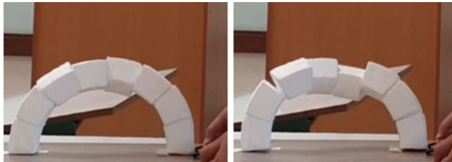
تصویر ۱۷: وقوع لغزش در زمان تناوب پایین در بلوک‌ها
