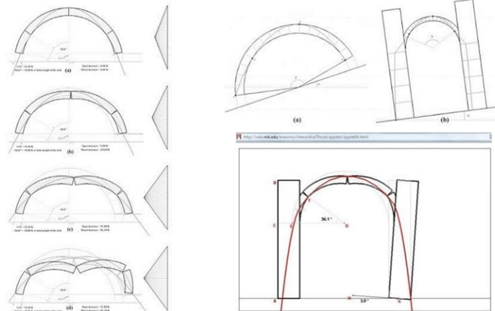
تصویر ۳: آموزش با تعامل دوسویه در دانشگاه ام. ای. تی. چاپ: تحلیل سینماتیک قوس، راست بالا؛ مدل سازی اثر زلزله، راست-پایین: اثر دوران پایه در نشست در پایداری سازه (Block et al 2006)
