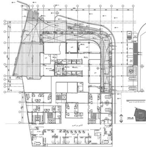
تصویر ۲: راست: پلان مبلمان طبقات ساختمان شهرداری مرکز؛ چپ: نمای بیرونی شهرداری مرکز
