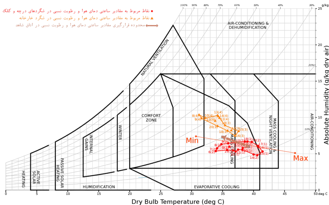
تصویر ۱۳: وضعیت دما و رطوبت نسبی روزهای مورد مطالعه برحسب مقادیر ساعتی به تفکیک تأثیر کلک و خارخانه بر روی نمودار سایکرومتریک گیوانی در دوره گرم سال (۱۸ تا ۲۱ تیر ۱۳۹۸)
