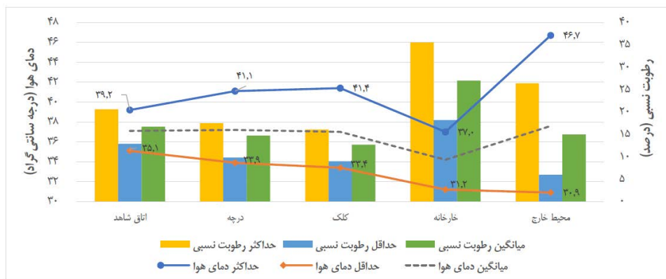
تصویر ۹: مقادیر حداقل، حداکثر و میانگین دمای هوا و رطوبت نسبی در بخش‌های مختلف بنا طی روزهای مورد مطالعه در دوره گرم سال
