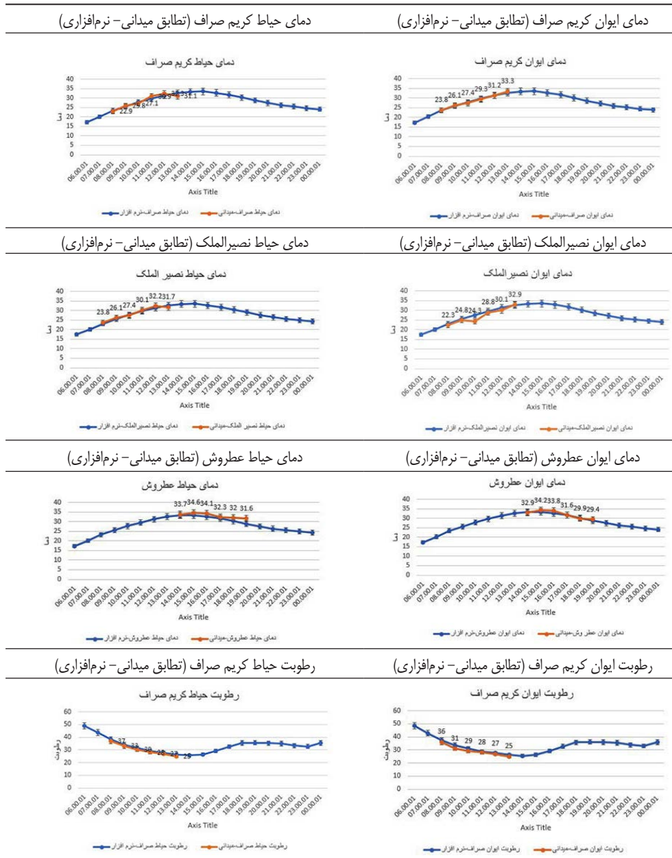
جدول ۶: مقایسه داده‌های نرم‌افزار با آزمایش میدانی
