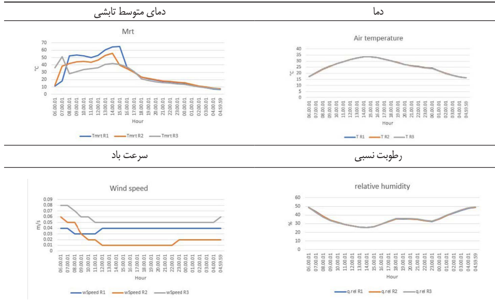
جدول ۱۳: نمودار داده‌های آب‌وهوایی خانه کریم صراف در سه رسپتور (R1 مرکز حیاط، R2 نزدیک ایوان و R3 مرکز ایوان)
