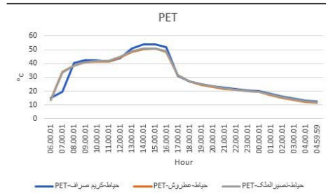
جدول ۲۴: نمودار آسایش حرارتی PET در حیاط سه خانه
