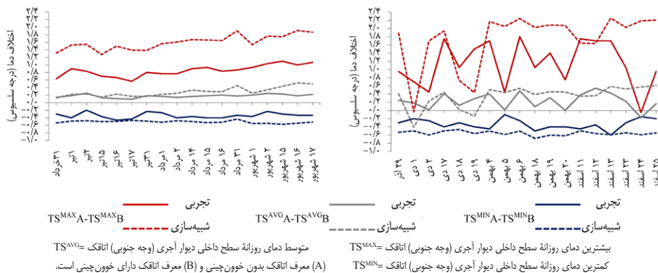
تصویر ۹: نمودارهای اختلاف بیشترین، کمترین و متوسط دمای روزانه سطح داخلی دیوار آجری (بدنه جنوبی) اتاقک‌ها در روزهای اندازه‌گیری تابستان (چپ) و زمستان (راست) ۱۳۹۸ با روش تجربی و شبیه‌سازی
