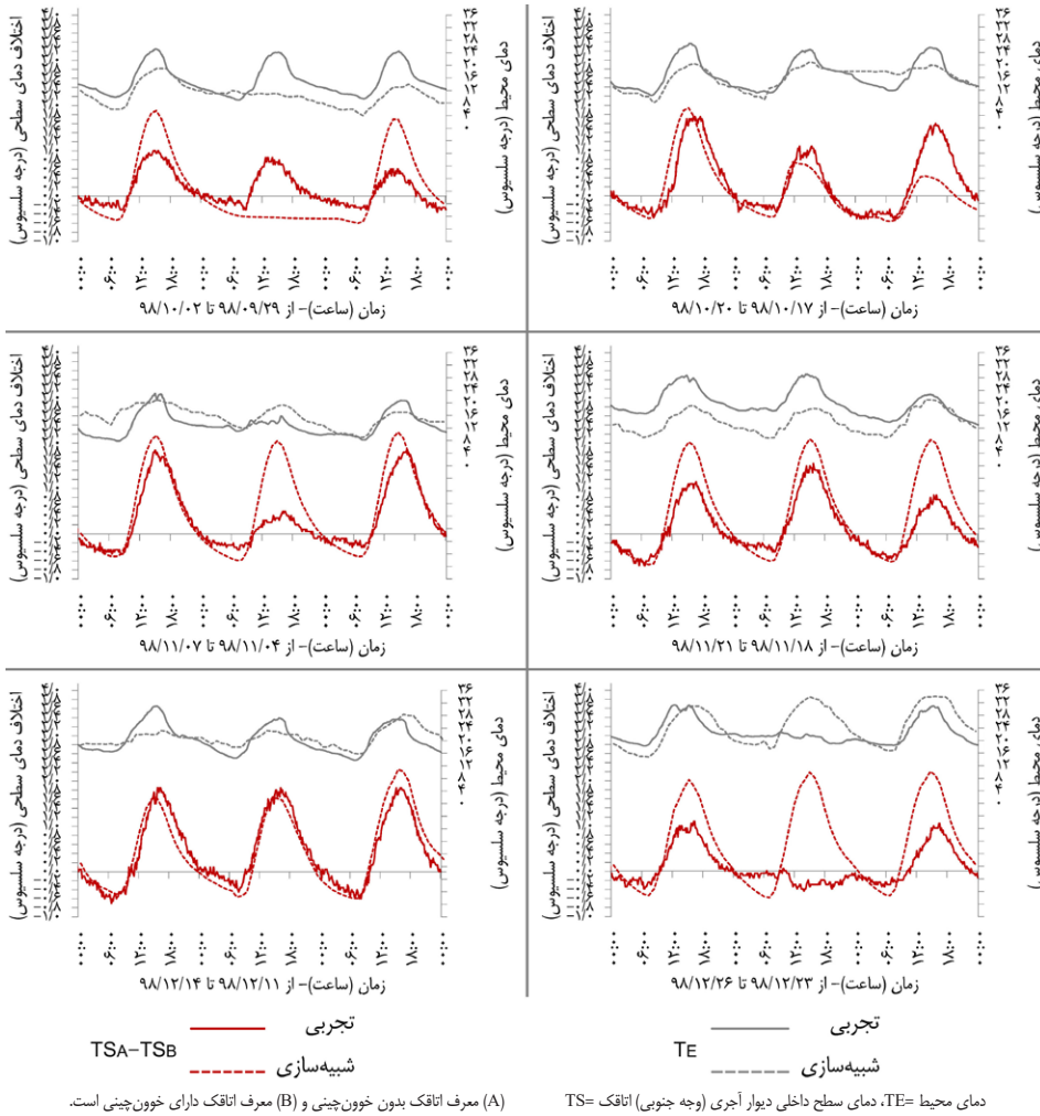
تصویر ۸: نمودار اختلاف میان دمای سطح داخلی دیوار آجری (بدنه جنوبی) دو اتاقک در دوره‌های اندازه‌گیری زمستان ۱۳۹۸ با روش تجربی و شبیه‌سازی
