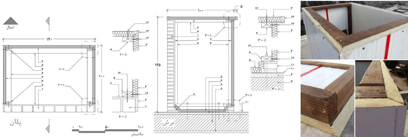
۱. دیوار آجری؛ ۲. پلاستر سیمان؛ ۳. ساندویچ پانل؛ ۴. چوب چهارتراش؛ ۵. کرسی آجری؛ ۶. عایق حرارتی پلی استایرن؛ ۷. بتن سبک؛ ۸. سازه سقف؛ ۹. اندود داخلی؛ ۱۰. پیچ ضدزنگ؛ ۱۱. ماهیچه بتنی؛ ۱۲. عایق رطوبتی با رویه آلومینیوم؛ ۱۳. ورق گالوانیزه
