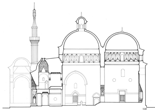
تصویر ۸: کارشیو مساجد گونه بورسا با ایوان‌های دارای پوشش گنبدخانه‌ای و یک نمونه تصویر و مقطع از اتصال گنبدخانه تالار مرکزی و فضای نمازخانه در مسجد یشیل بورسا. کارشیوها به ترتیب: اورخان قاضی (۷۴۰ق)، ایلدیریم بایزید (۷۹۸ق)، یشیل (۸۲۲-۸۲۴ق)، سلطان مراد دوم (۸۵۴ق) در بورسا و مسجد مرادیه ادرین (۸۳۹ق) (Freely 2011).
