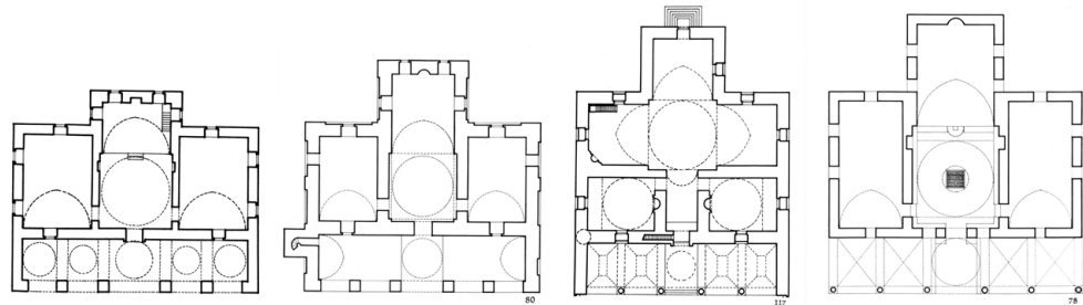
تصویر ۷: کارشیو برخی از مساجد گونه بورسا که فضای نمازخانه دارای طاق آهنگ است. به ترتیب: مسجد سلطان اورخان قاضی در ازینق (۷۳۴ق)، مسجد خداوندگار در ادرین (اواسط قرن ۸ق)، مسجد ابواسحاق کارزونی (اواخر قرن ۸ق) و مسجد تیمورتاش در بورسا (Freely 2011).
