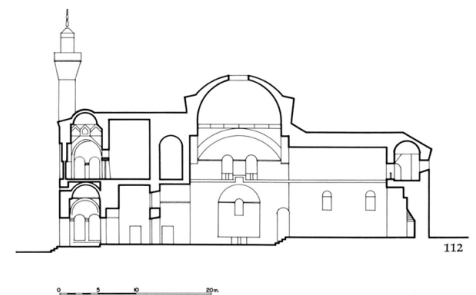
تصویر ۶: کارشیو، مقطع و تصویری از مسجد خداوندگار بوسا (۷۸۷ق) که چهار ایوان اطراف میان‌سرای گنبددار، دارای طاق آهنگ هستند (Freely 2011).
