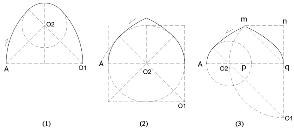
تصویر ۳: روش ترسیم قوس‌ها و شماره‌گذاری آن‌ها. (۱) قوس تخم‌مرغی. (۲) قوس مربع (پاتو پا - نیزه‌ای). (۳) پنج و هفت تند. جهت حرکت ریسمان در ترسیم هر قوس نشان داده شده است.
