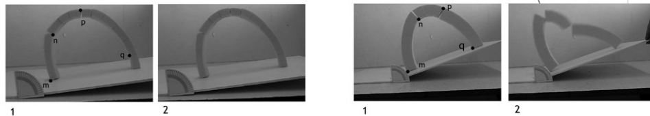
تصویر ۱۴: بررسی فروریختگی قوس شماره ۱ با تحلیل خط رانش، مشخص کردن زاویه دوران، شتاب افقی (a) و محل مفاصل پلاستیک. (بالا - چپ: برای نسبت ضخامت به دهانه ۱/۱۰. بالا-راست: برای نسبت ضخامت به دهانه ۲/۱۰). مراحل ۱ و ۲، محل و لحظه تشکیل مفاصل پلاستیک و فروریختگی در مدل فیزیکی می‌باشند. (پایین-چپ: برای نسبت ضخامت به دهانه ۱/۱۰. پایین-راست: با نسبت ضخامت به دهانه ۲/۱۰)
