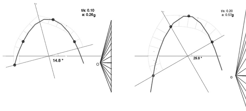
تصویر ۱۴: بررسی فروریختگی قوس شماره ۱ با تحلیل خط رانش، مشخص کردن زاویه دوران، شتاب افقی (a) و محل مفاصل پلاستیک. (بالا - چپ: برای نسبت ضخامت به دهانه ۱/۱۰. بالا-راست: برای نسبت ضخامت به دهانه ۲/۱۰). مراحل ۱ و ۲، محل و لحظه تشکیل مفاصل پلاستیک و فروریختگی در مدل فیزیکی می‌باشند. (پایین-چپ: برای نسبت ضخامت به دهانه ۱/۱۰. پایین-راست: با نسبت ضخامت به دهانه ۲/۱۰)
