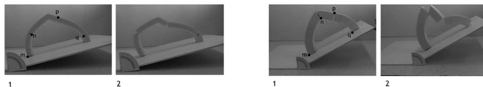
تصویر ۱۵: بررسی فروریختگی قوس شماره ۲ با تحلیل خط رانش، مشخص کردن زاویه دوران، شتاب افقی (a) و محل مفاصل پلاستیک. (بالا - چپ: برای نسبت ضخامت به دهانه ۱/۱۰. بالا-راست: برای نسبت ضخامت به دهانه ۲/۱۰). مراحل ۱ و ۲، محل و لحظه تشکیل مفاصل پلاستیک و فروریختگی در مدل فیزیکی هستند. (پایین-چپ: برای نسبت ضخامت به دهانه ۱/۱۰. پایین-راست: با نسبت ضخامت به دهانه ۲/۱۰) ۳۲
