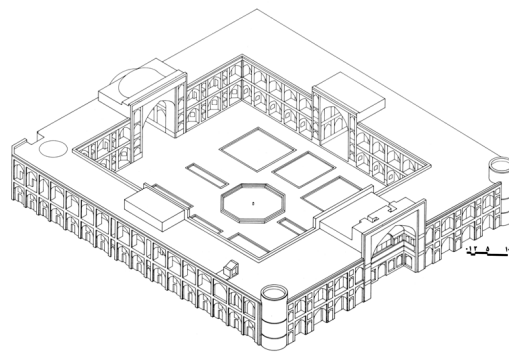
تصویر ۲: راست: مرکزیت در مدارس، تصویر سه بعدی مدرسه خان شیراز که الگوی چهار ایوانی در آن دیده می‌شود، اثر مربوط به دوره صفوی و طراح آن استاد حسین شماعی است (وزارت مسکن و شهرسازی ۱۳۸۸، ۳۱). چپ: مرکزیت بازار در شهر تبریز، بازار تبریز در دوره قاجاریه (همان، ۴۷).
