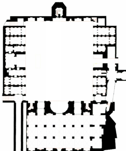
تصویر ۱۹: پلان مسجد عمادالدوله کرمانشاه (انسان سازمان میراث فرهنگی کرمانشاه)
