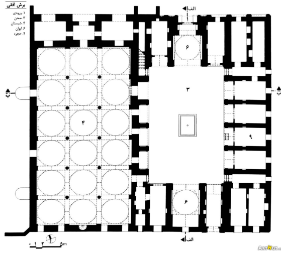
تصویر ۱۴: پلان مسجد جامع مهاباد (حاجی قاسمی ۱۳۸۳)
