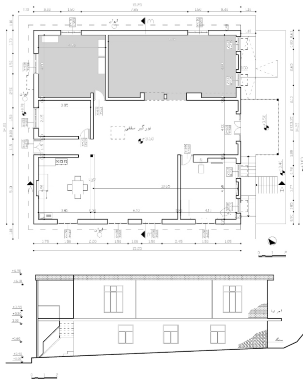
تصویر ۴: پلان و نمای ساختمان موجود
