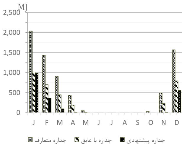
نمودار ۱: بار گرمایی مدل نمونه در صورت استفاده از ۳ نوع جدار مورد بررسی
