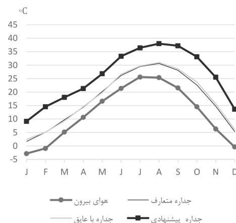
نمودار ۳: میانگین ماهانه دمای هوای بیرون و اتاق در سه حالت جدار متعارف، باعایق و پیشنهادی
