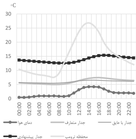
نمودار ۴: نوسان دمای ساعتی در روز ۲۱ دسامبر (اول دی)
