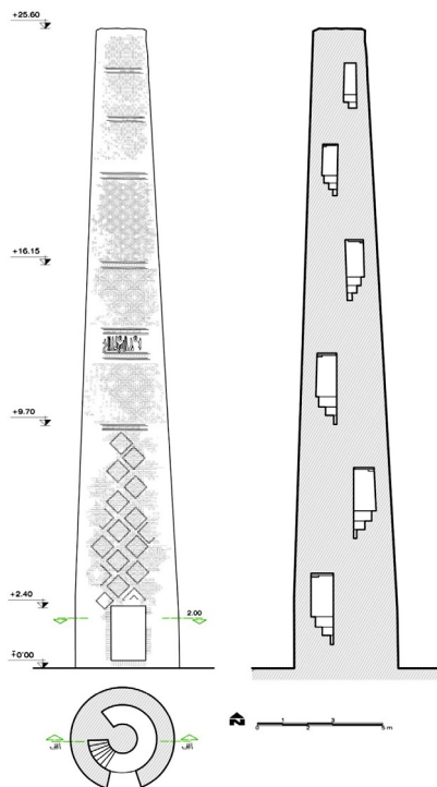
تصویر ۲۵: برش افقی و عمودی و نمای منار تاریخانه دامغان از سه تراز مختلف (برداشت و ترسیم محمد بلوری همان ۱۰۷)
