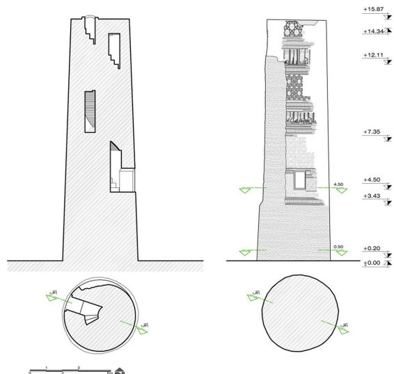
تصویر ۳۱: نقشه‌های منار مسجد جامع ساوه، گوشه‌ای از تزئینات، (منبع: هفت خشت پارس، ویرایش میترا آزاد، محمد بلوری)
