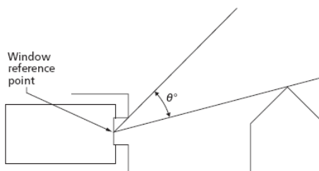
تصویر ۱۱ - زاویه دید آسمان
