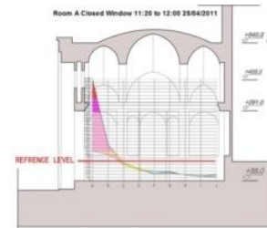
تصویر ۴- نمودارهای هم‌روشنایی روی پلان (تصویر چپ) و برش قائم (تصویر راست) اتاق A از خانه عمری ها در روز ۵ اردیبهشت ۱۳۹۰
