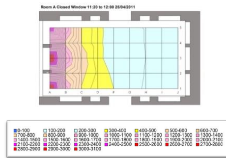
تصویر ۴- نمودارهای هم‌روشنایی روی پلان (تصویر چپ) و برش قائم (تصویر راست) اتاق A از خانه عمری ها در روز ۵ اردیبهشت ۱۳۹۰
